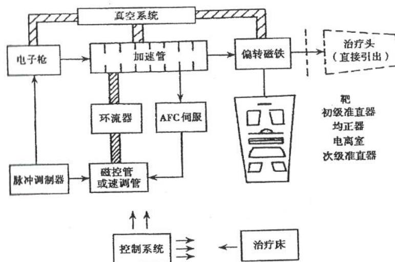
图 9-2 典型的直线加速器的结构系统图
