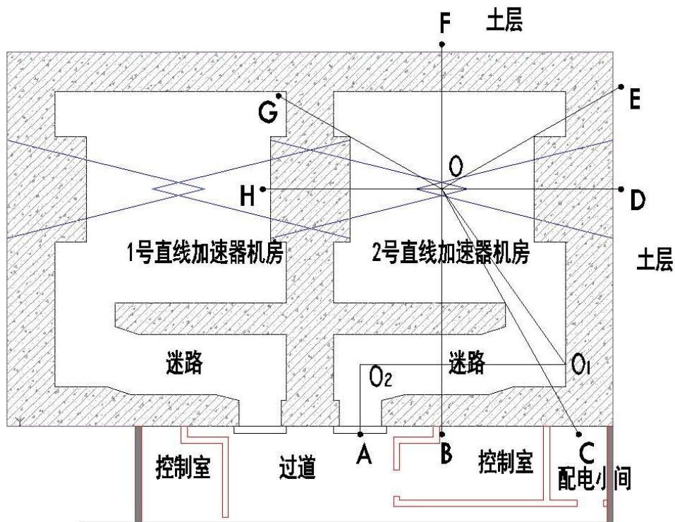
图 11-1 加速器机房平面布置图（单位：mm）
