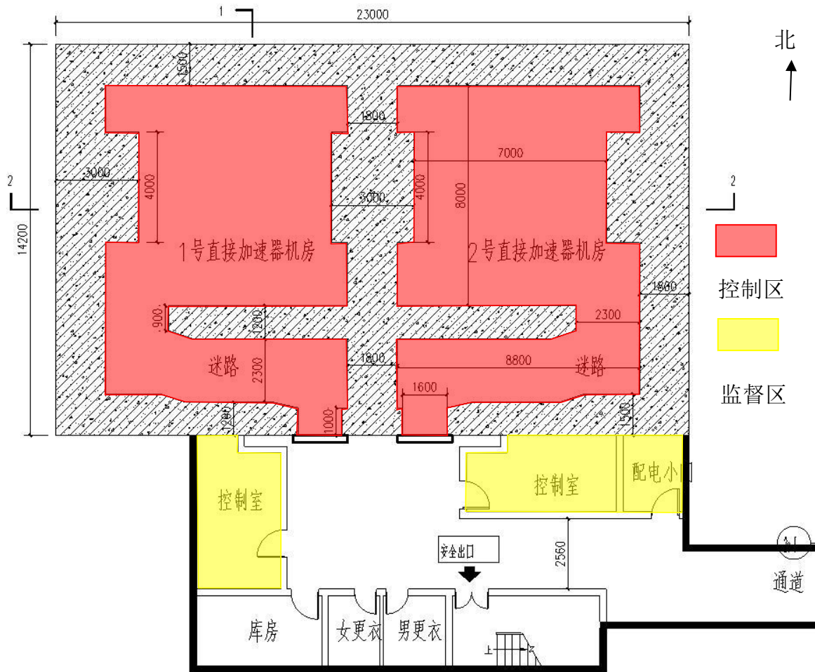
图 10-1 2间直线加速器机房平面图（单位：mm）
