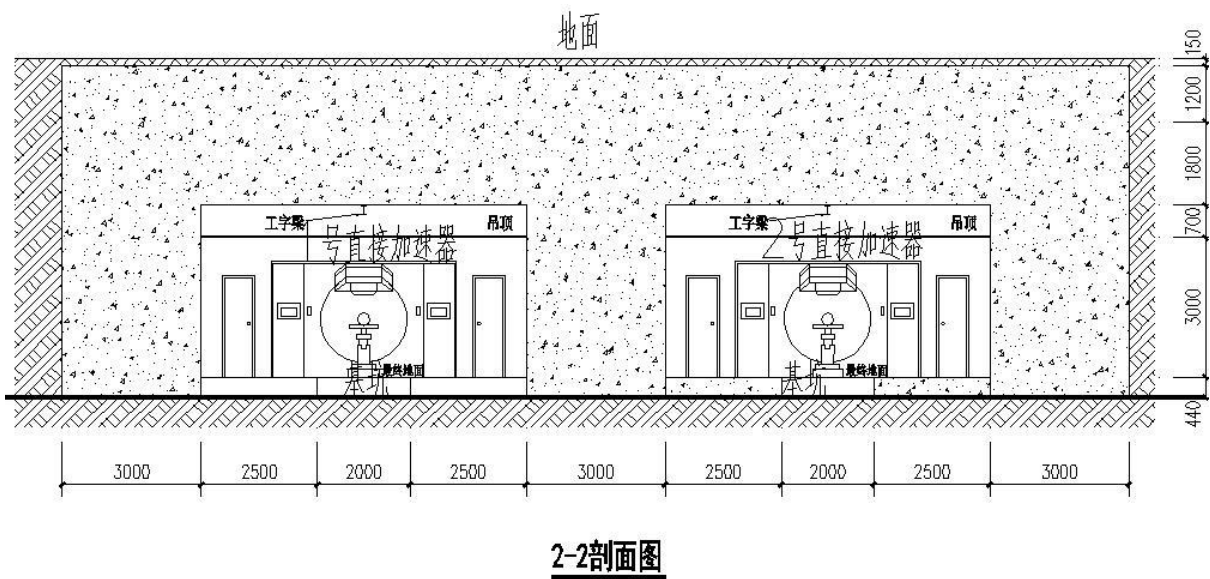
图 10-3 加速器机房 2-2 剖面图（单位：mm）
