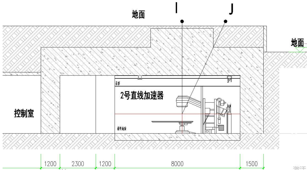
图 11-2 加速器机房剖面图（单位：mm）
