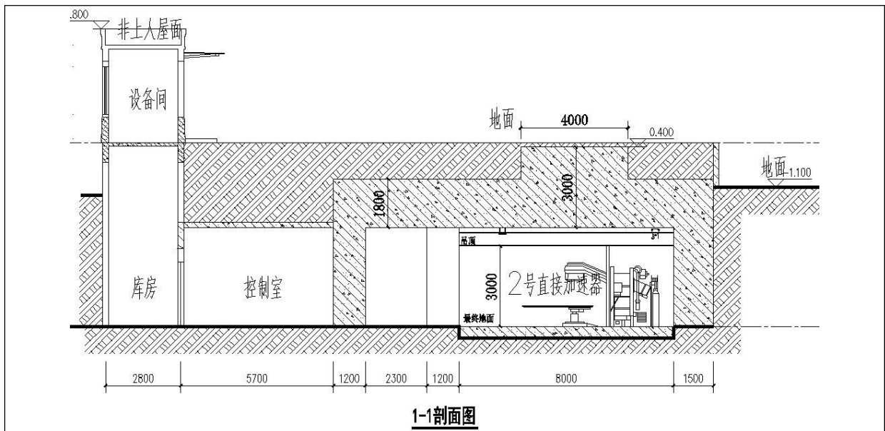
图 10-2 加速器机房 1-1 剖面图（单位：mm）
