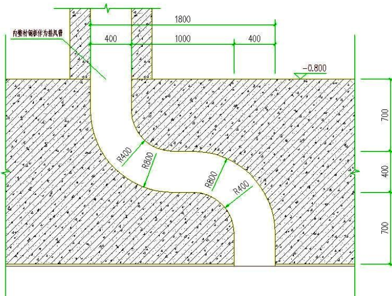
图 10-5 加速器机房分管布置图
