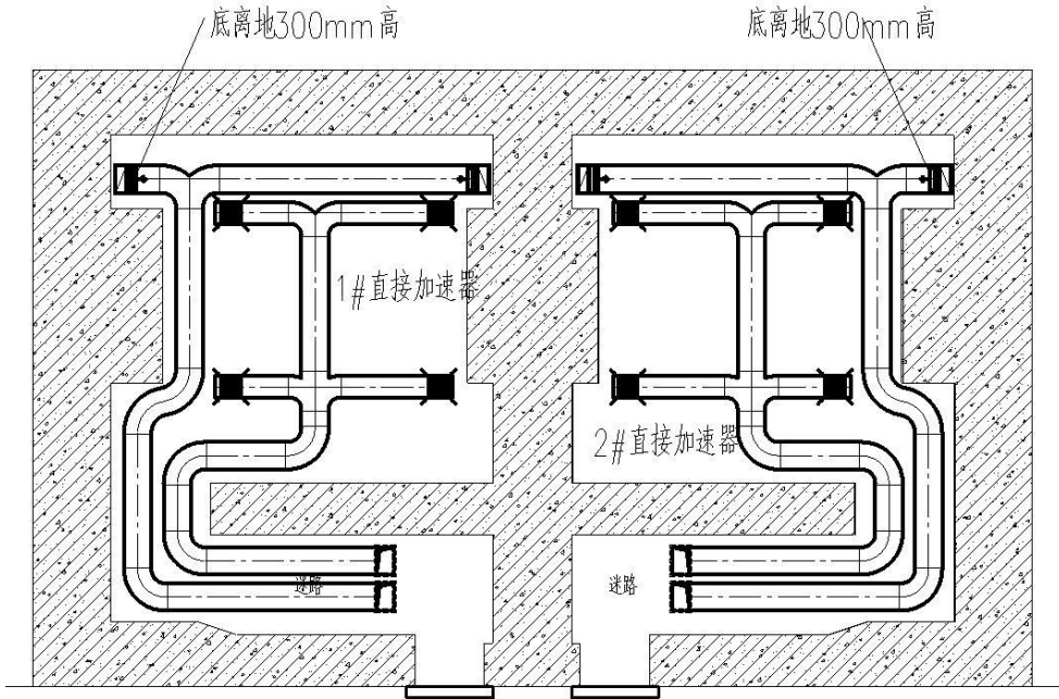
图 10-5 加速器机房分管布置图
